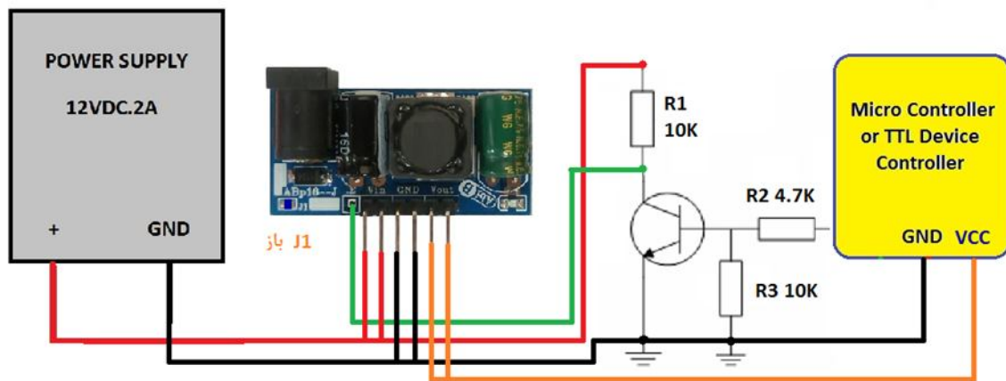
شکل 3: راه اندازی مبدل ABp163BJ-C با پین فعال ساز
