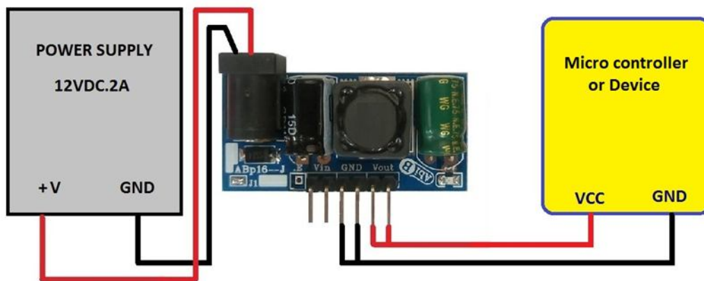
شکل 2: راه اندازی مبدل ABp163BJ-C بدون پین فعال ساز
