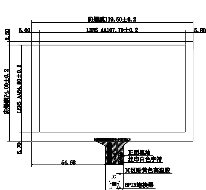
正视图
