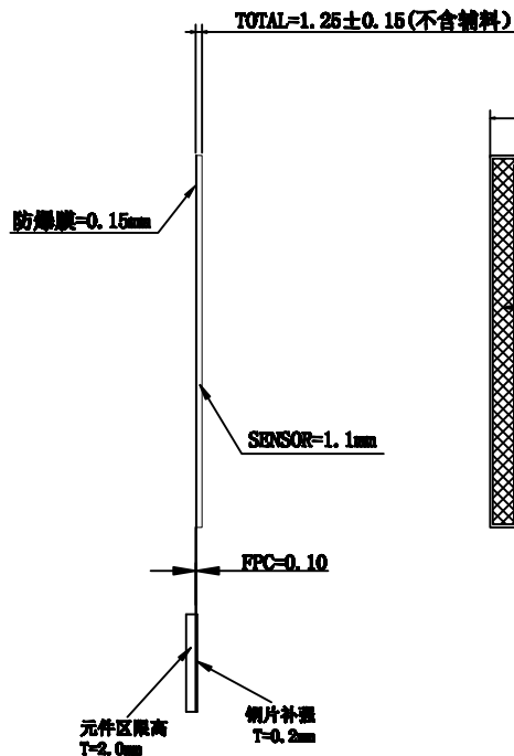
侧视图
