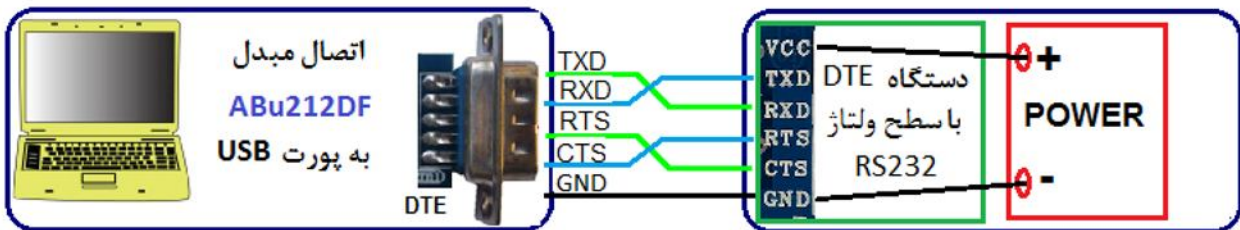
- اتصال Cross مبدل به دستگاه DTE با سطح ولتاژ RS232 به همراه Handshaking
