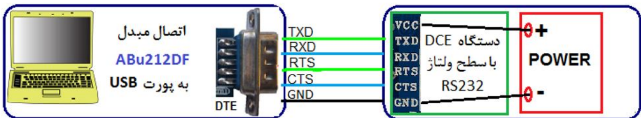
- اتصال Straight مبدل به دستگاه DCE با سطح ولتاژ RS232 به همراه Handshaking
