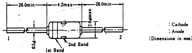
(JEDEC DO-35)
