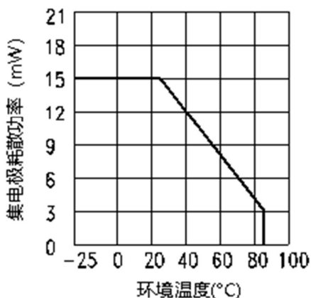
图三：耗散功率VS环境温度曲线
