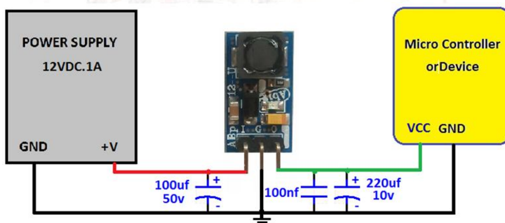
شکل 1: راه اندازی و اتصال خازنهای خارجی مبدل ABp122CU
