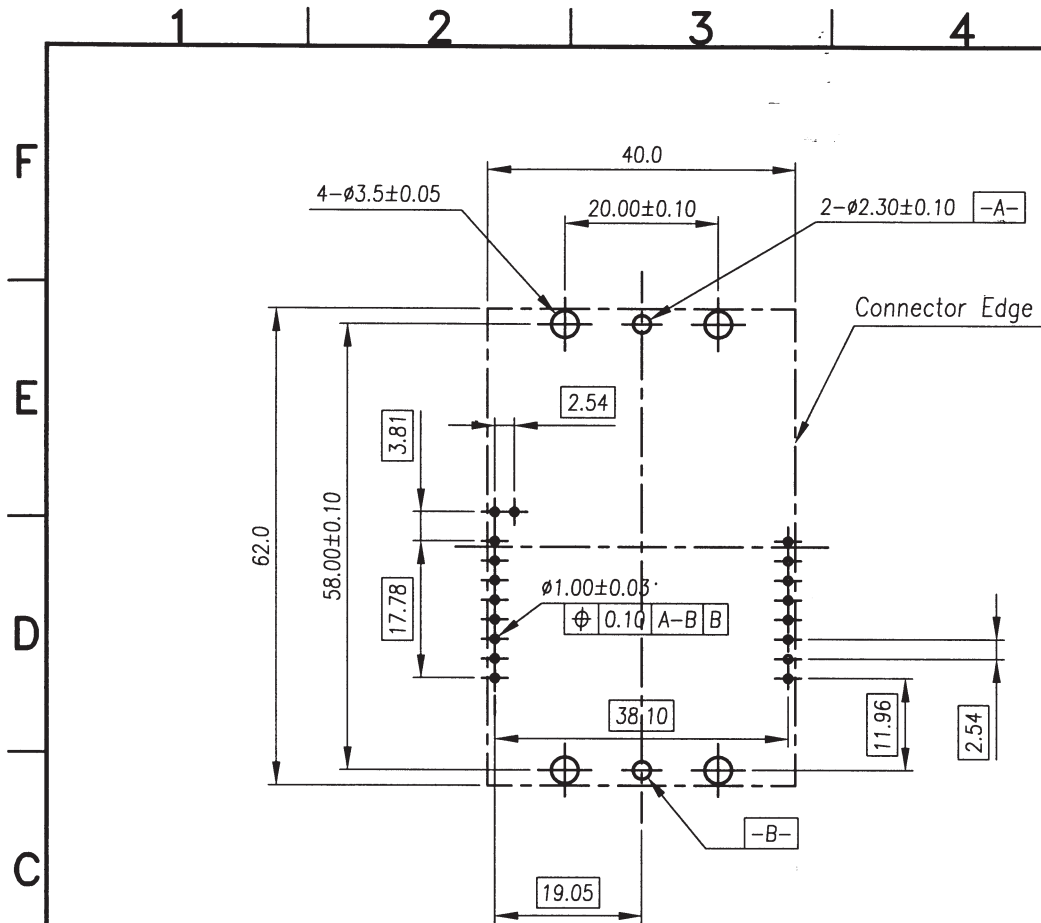
P.C.B. Layout
