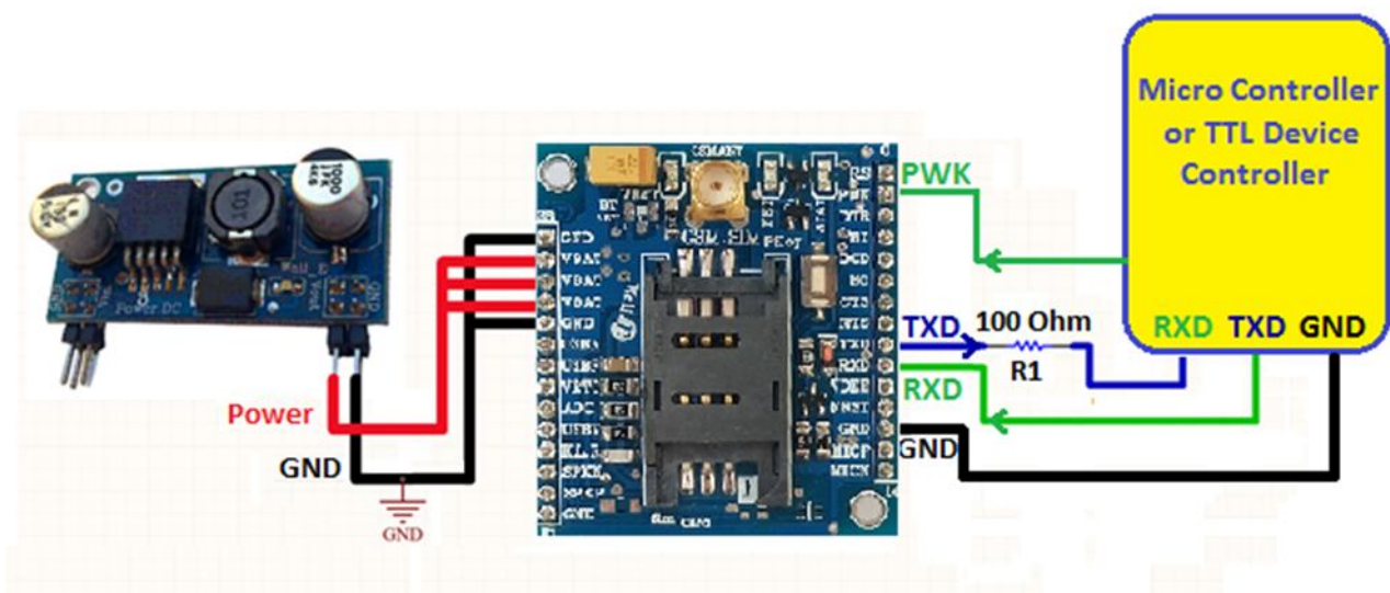
شکل 4: اتصال توسعه ABg131S به میکروکنترلر
