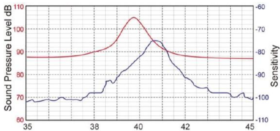
图 3: 声压灵敏度
