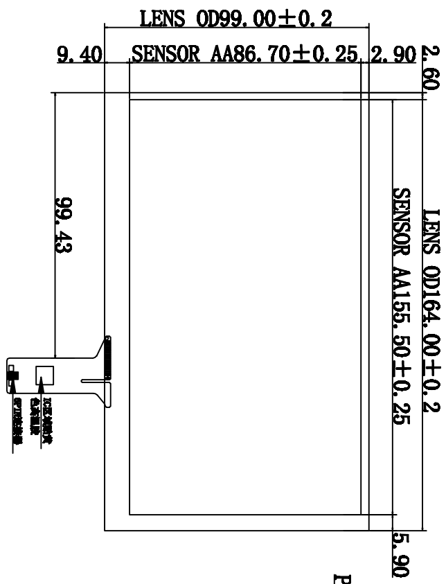
正视图
