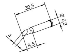
0102BDLF20/SB PLCC blade
