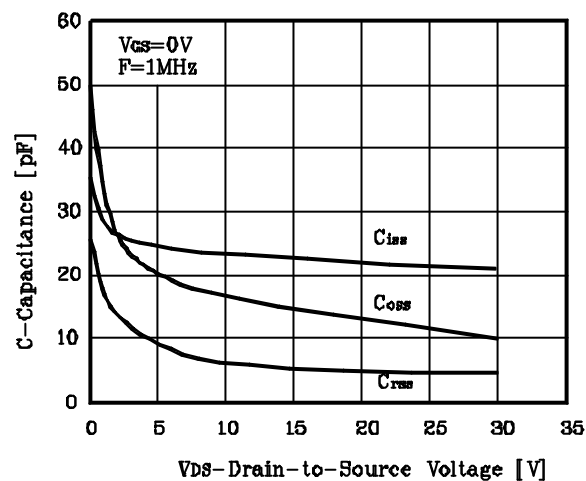
Fig. 4 C - V_{DS}
