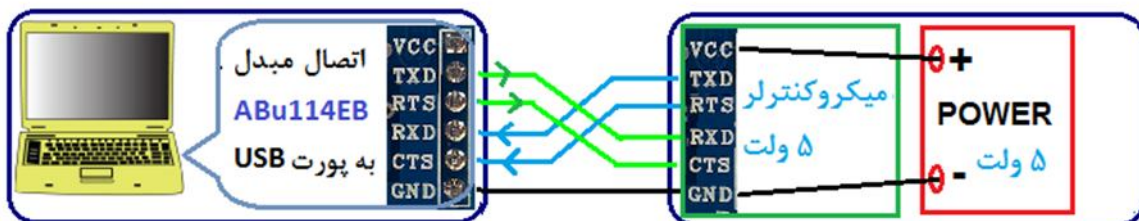
- اتصال مبدل با جامپر +5 به دستگاه با سطح ولتاژ منطقی TTL به همراه Handshaking
