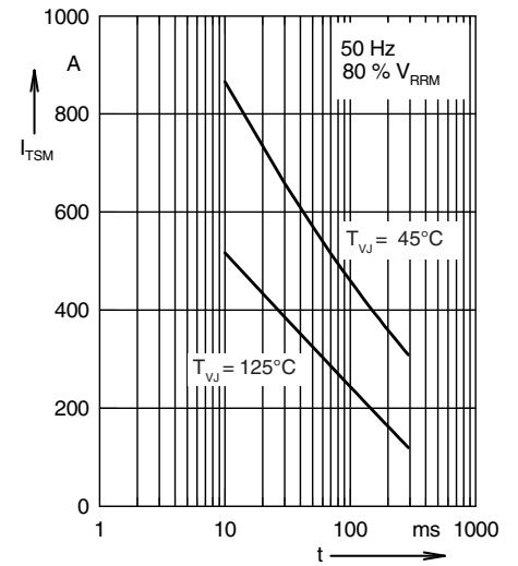
I_{TSM} , I_{FSM} : Crest value, t : duration
