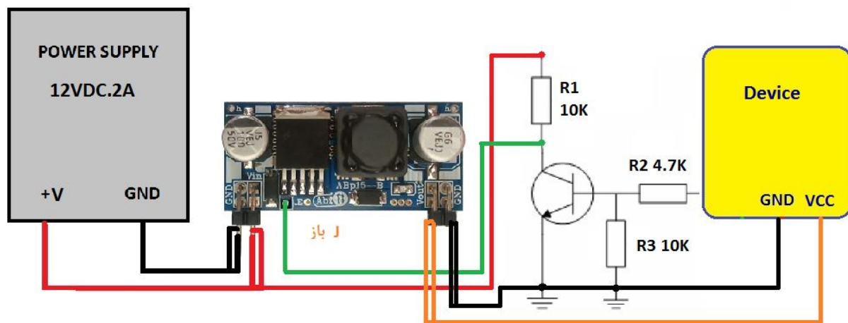
شکل 2: راه اندازی مبدل ABp153BB-C با پین فعال ساز
