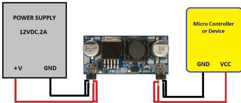
شکل 2: راه اندازی مبدل ABp153BB-C بدون پین فعال ساز
