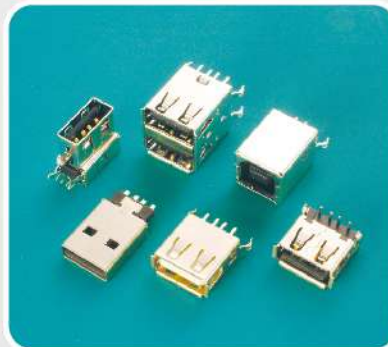
USB (1.1 and 2.0) ■ A/B Type ■ Plug/Receptacle ■ DIP/SMT type
