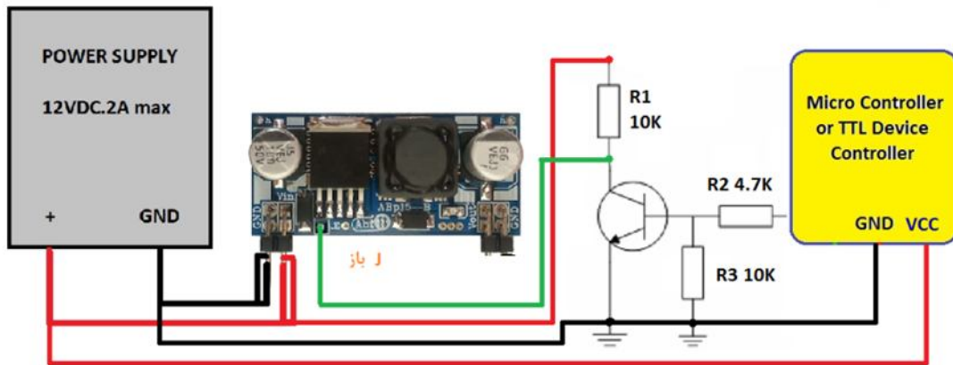
شکل 2: راه اندازی مبدل ABp15gBB-C با پین فعال ساز
