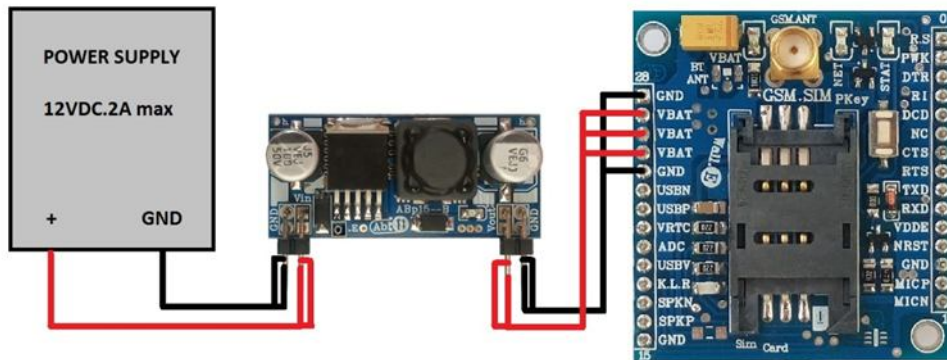
شکل 1: اتصال مبدل ABp15gBB-C به جی اس ام
