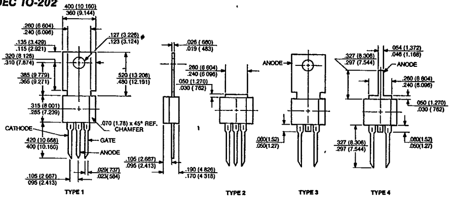
JEDEC TO-202
