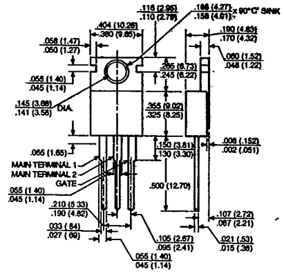
JEDEC TO-220AB
