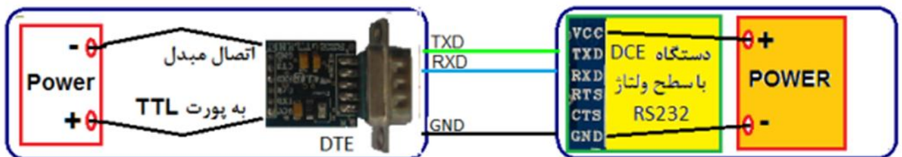
- اتصال Straight مبدل به دستگاه DCE با سطح ولتاژ RS232
