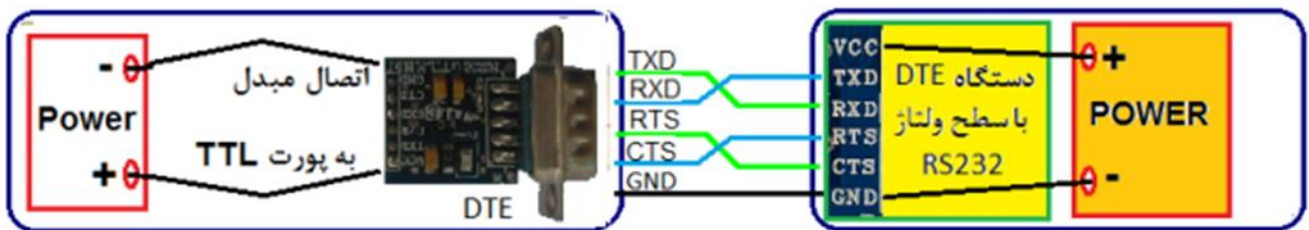
- اتصال Cross مبدل به دستگاه DTE با سطح ولتاژ RS232 به همراه Handshaking
