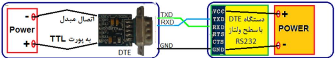
- اتصال Cross مبدل به دستگاه DTE با سطح ولتاژ RS232
